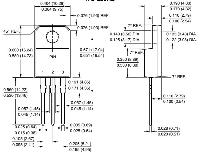
ITO-220AB
