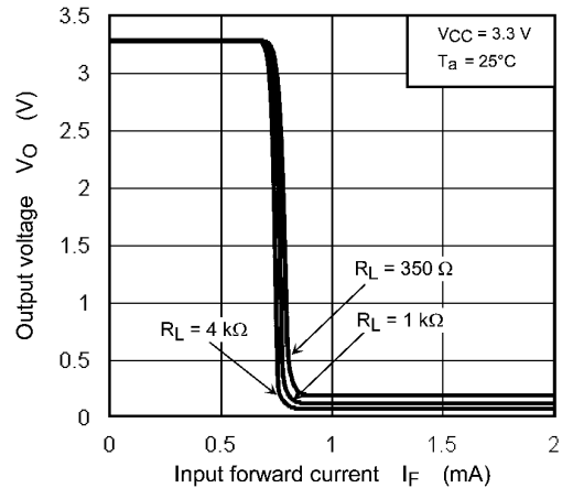
Fig. 12.2.6 V_O - I_F
