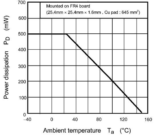
Fig. 7.14 P_D - T_a
