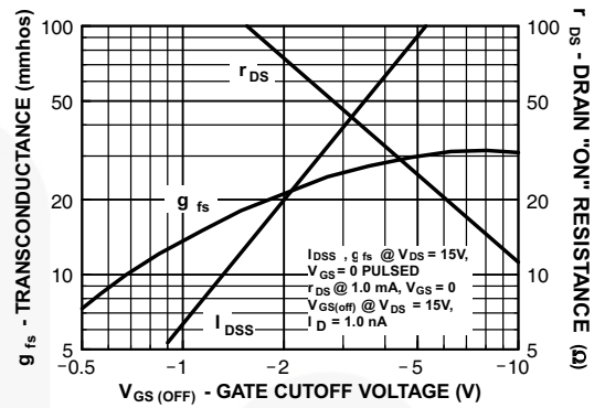
Figure 4. Parameter Interactions
